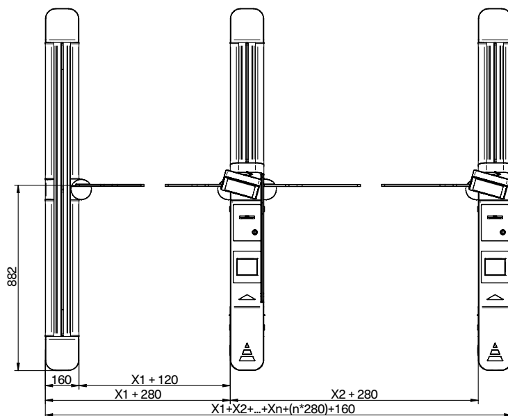
mPass (2-Linien-Konfiguration) – Ansicht von oben
