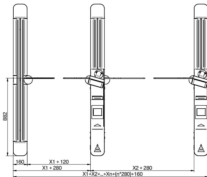
mGo (configuración de 2 vías) – vista superior
