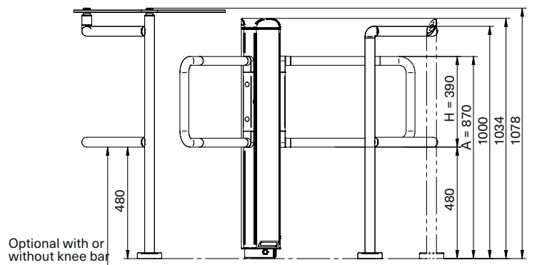
mTwing con barras en U – vista lateral
