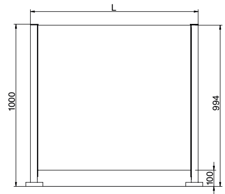
mGuide vista desde delante
