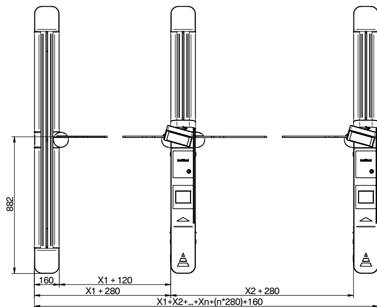
mPass (configuration 2 lignes) – vue de dessus
